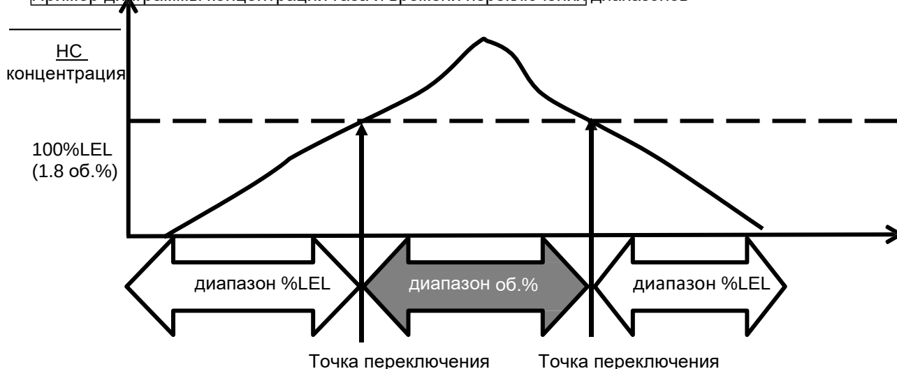
Пример диаграммы концентраций газа и времени переключения диапазонов
